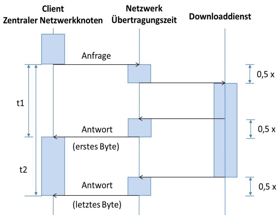
Abbildung 5: QoS Netzwerkdigramm
